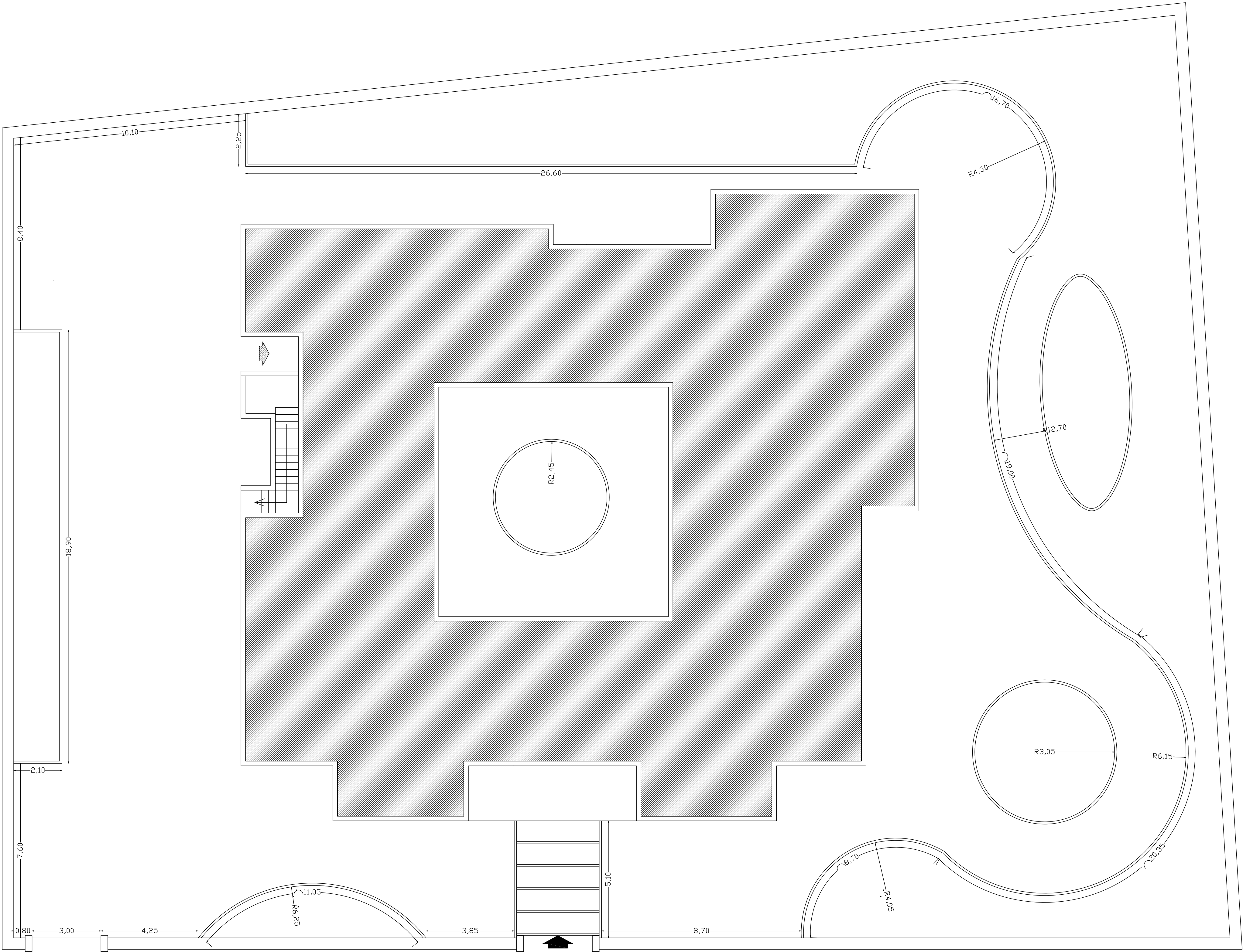
PLANIMETRIA QUOTATA scala 1:100
